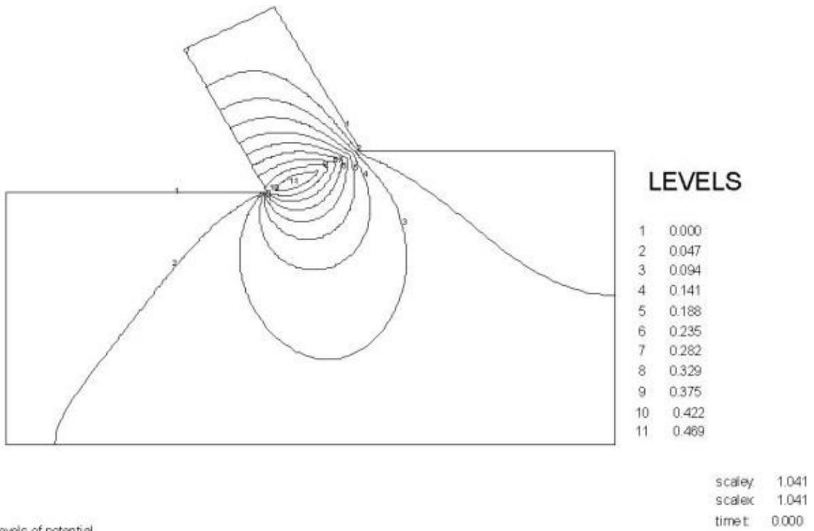
Figure S-3: The equipotential lines.
