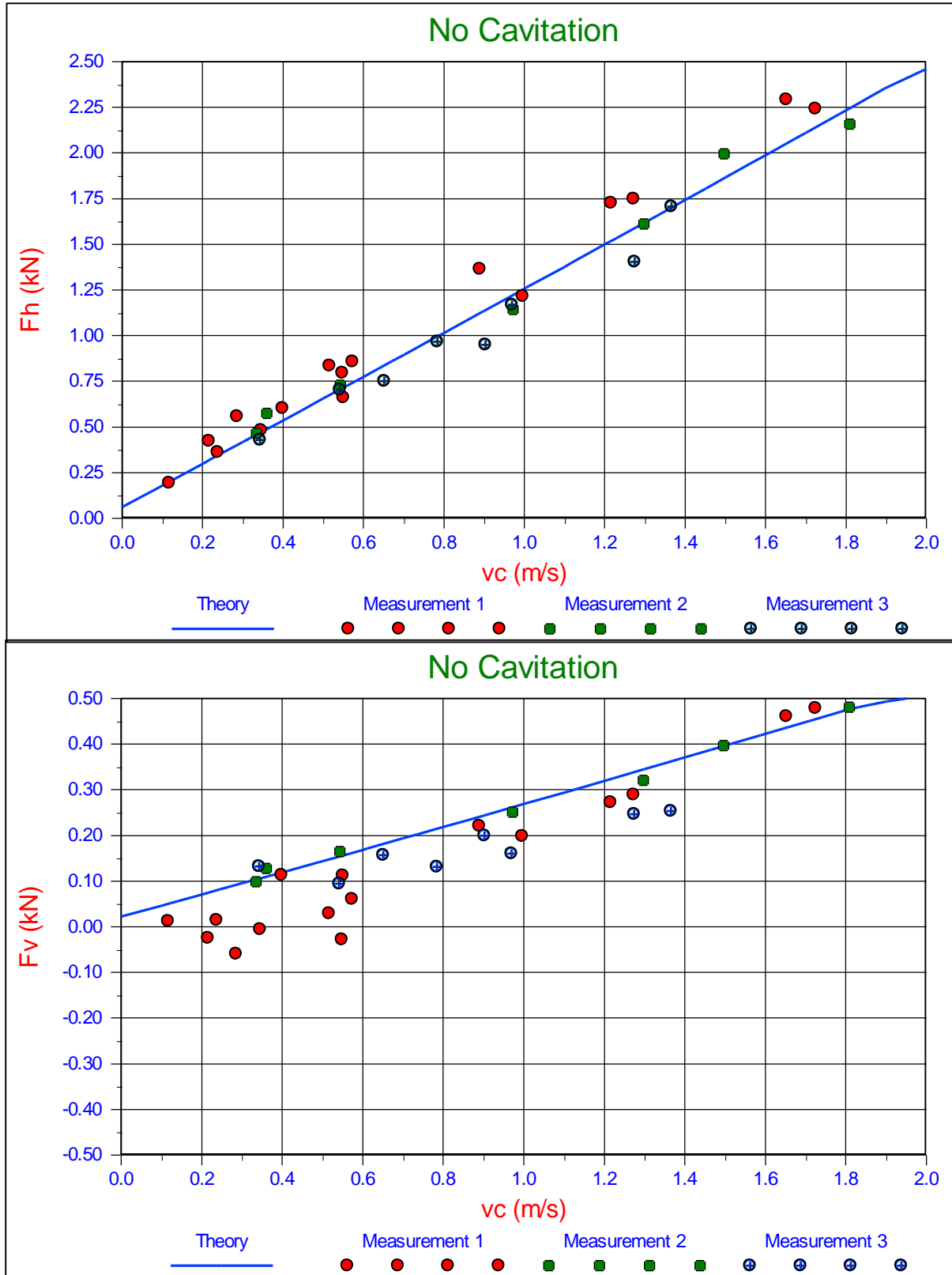
Figure M-23: \alpha=45^\circ , h_i=47 mm, h_b=141 mm.
