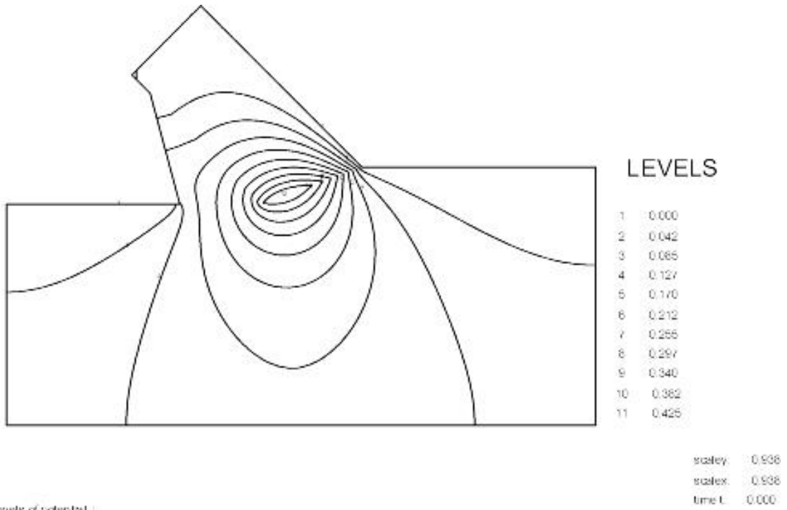
Figure S-10: The equipotential lines.
