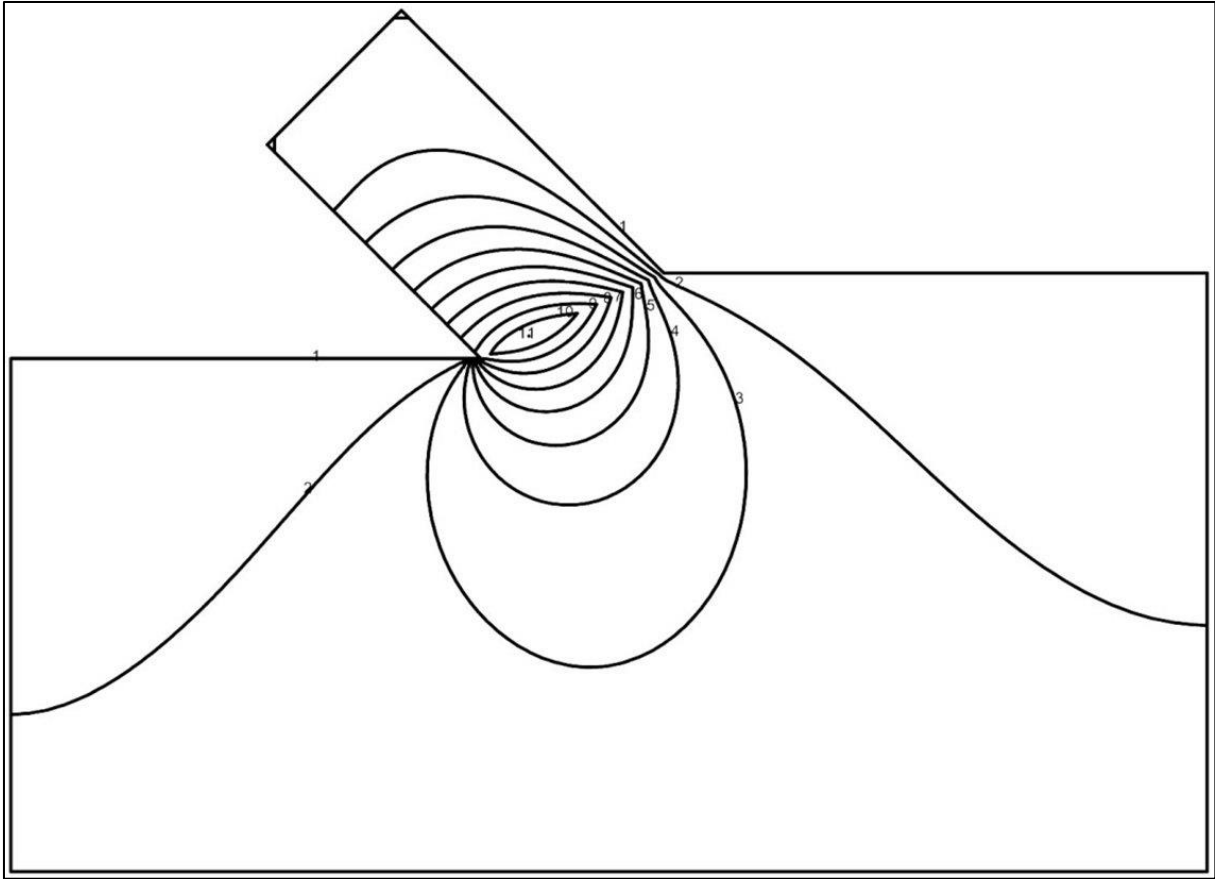
Figure 6-14: The equipotential lines.
