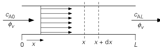
Figuur 1.7. Een propstroomreactor
